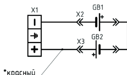
Рис. 5.2. Схема электрическая соединения АКБ в линейку для БК 1000 ВА (2 АКБ, 24 В)
